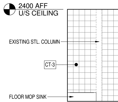
5 UTR 107 - West A104/A702 1:50
